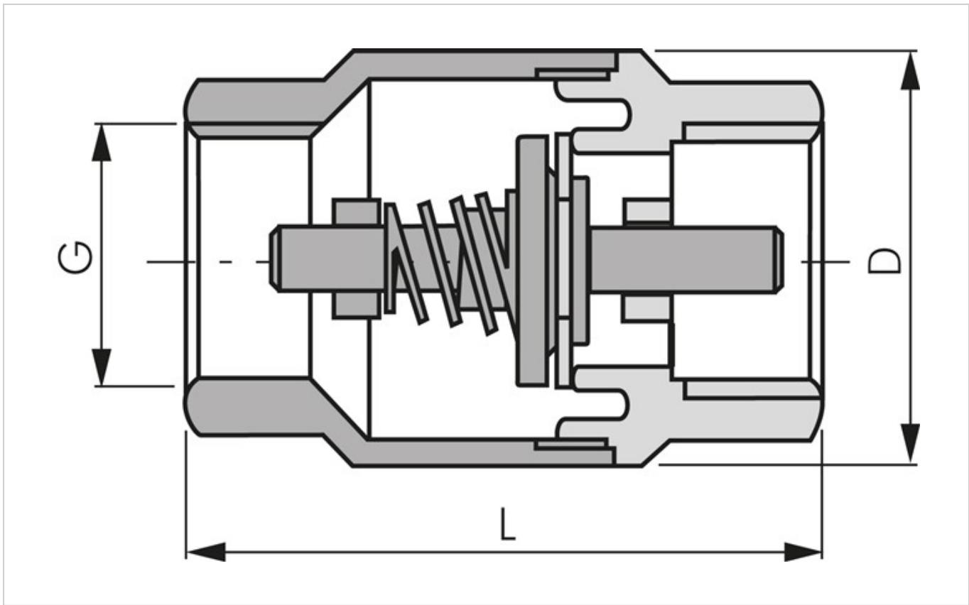
Zeichnung: Rückschlagventil
