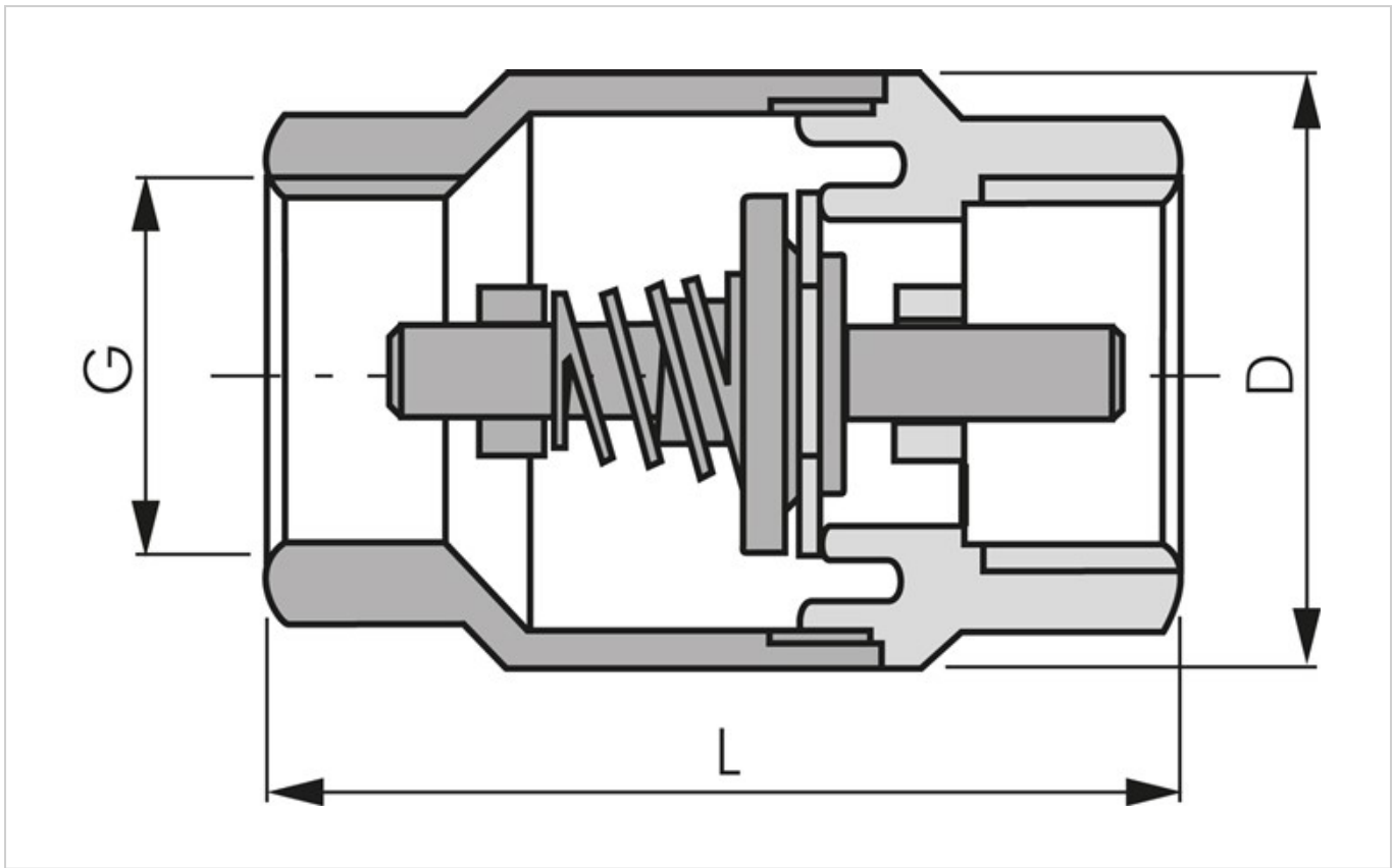
Drawing: Rückschlagventil
